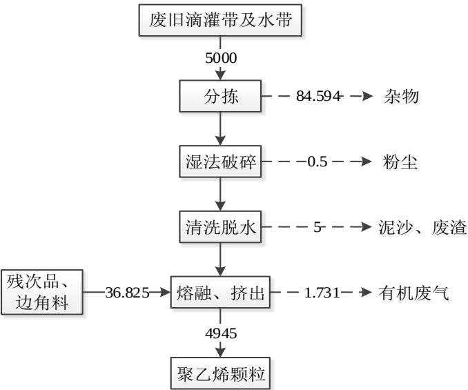
图 3.2-3 造粒生产线物料平衡图 单位: t/a
